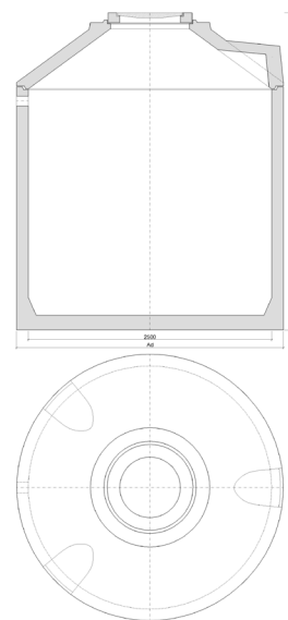
Güllebehälter DN 2500
