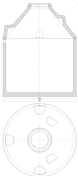
Güllebehälter DN 2400
