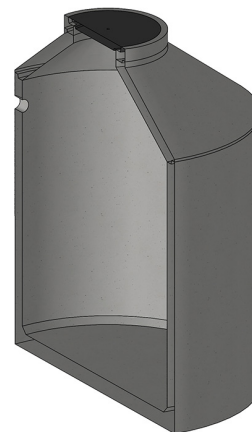
Güllebehälter DN 2500
